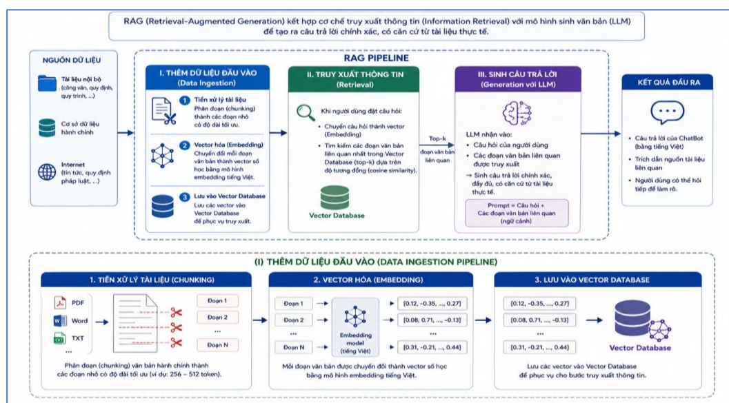
Hình 3: Kiến trúc RAG của hệ thống ChatBot AI hành chính
